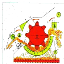
Рис. 27 Молотильный аппарат комбайна «ДОН-1500»: 1 — молотильный барабан; 2 — молотильный транспортер; 3 — молотильный барабан; 4 — подбарабан; 5 — молотильный барабан
